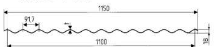
МП18-1100
