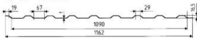
C17-1090 ТУ 1122-079-02494680-01
